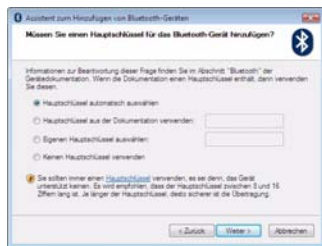
Abb. 23 - Hauptschlüssel-Option
