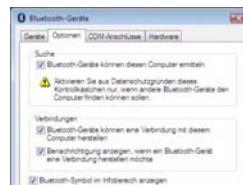
Abb. 24 Bluetooth-Geräte- Optionen
