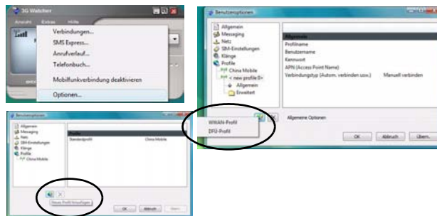
Abb. 14 - WWAN-Profil hinzufügen
