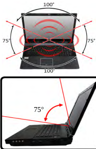
Figura 12 - Emisor - Ángulos de visión
