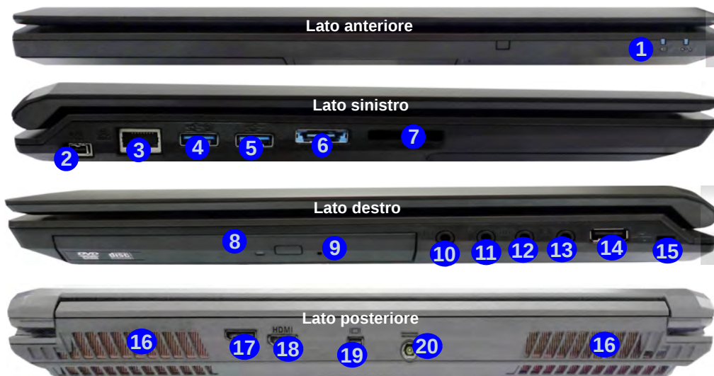
Figura 9 - Vista anteriore, sinistra, destra e posteriore (Modelli A & C)
